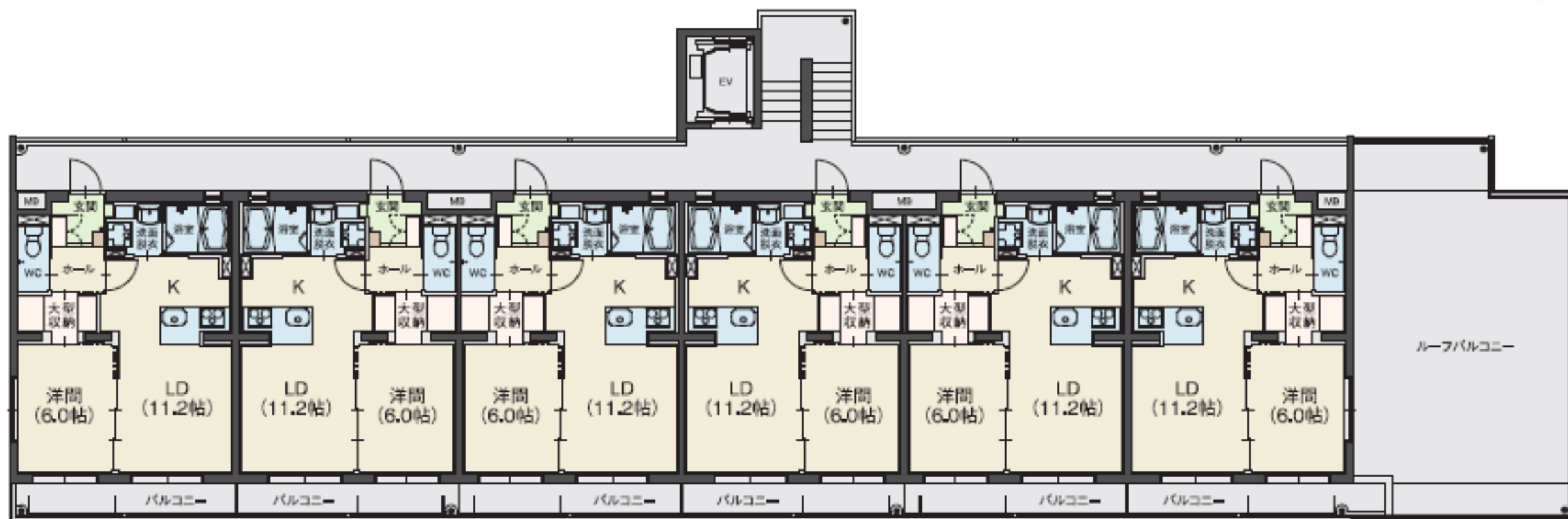
5階平面図
